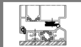
hliníkový podlahový práh s PTM (20 mm)
